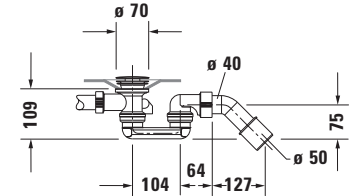
Siphon für Badewanne # 700449
