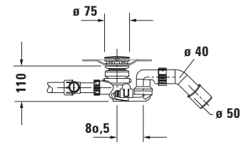
Siphon mit Bodenzulauf für Whirlwanne # 760451
