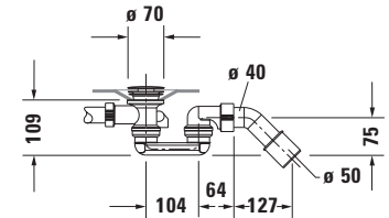
Siphon für Badewanne # 700451
