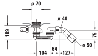
Siphon für Badewanne # 700453
