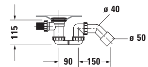
Siphon für Whirlwanne # 760449
