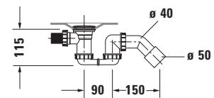
Siphon für Whirlwanne # 760450
